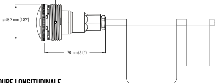
COUPE LONGITUDINALE
